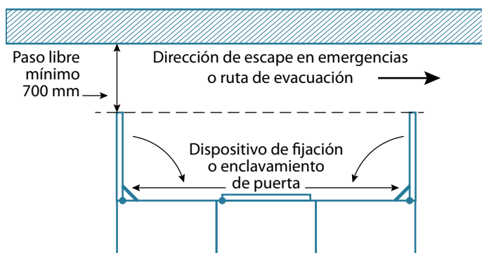
Figura 9. Pasillo, pasos libres mínimos
