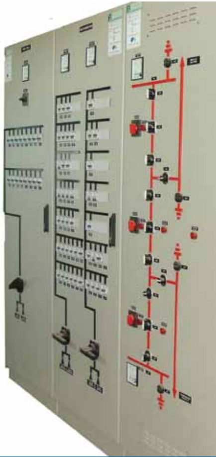
Figura 2. Gabinete fijado al piso
