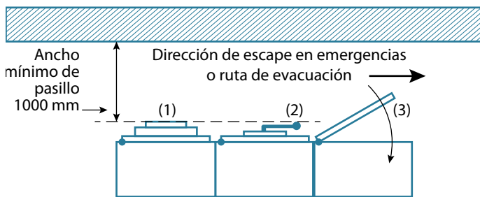
Figura 7. Pasillo, ancho mínimo
