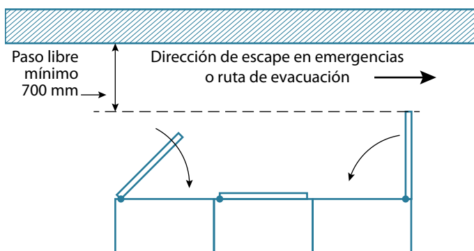
Figura 10. Pasillo, paso libre mínimo
